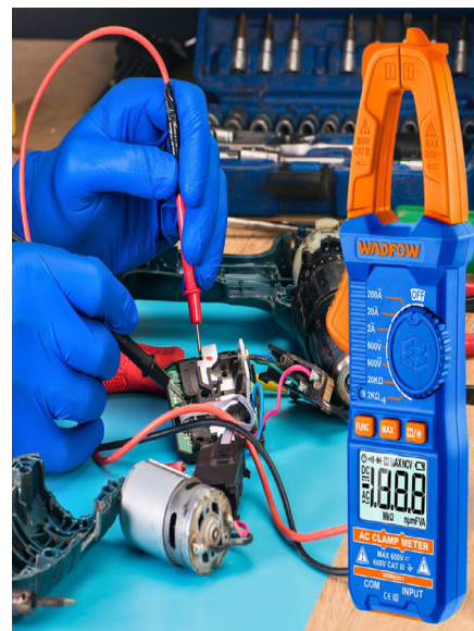
PINZA AMPERIMÉTRICA DIGITAL-WDM6501
