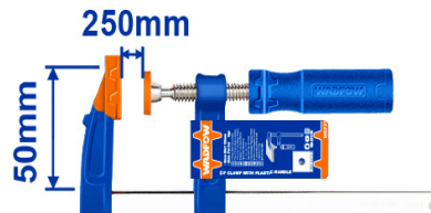
PRENSA F CON MANGO DE PLÁSTICO-WCP2153
