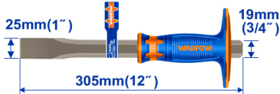
CINCEL PARA CONCRETO-WCC2312
